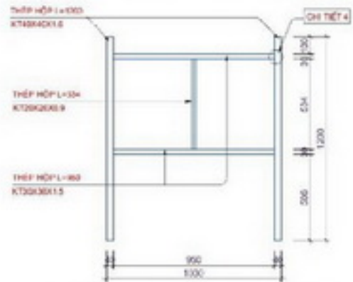
MẶT ĐỨNG KHUNG A TL 1/25
