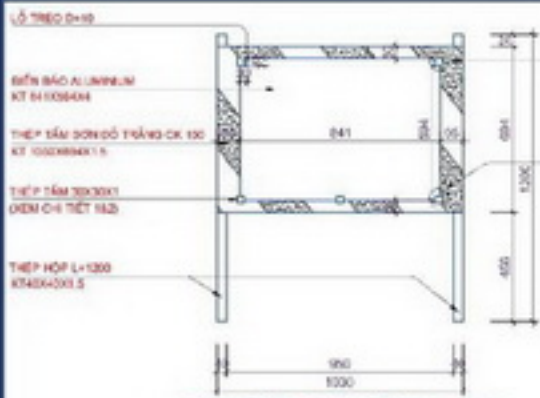
MẶT ĐỨNG TRƯỚC TL 1/25
