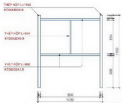
MẶT ĐỨNG KHUNG B TL 1/25
